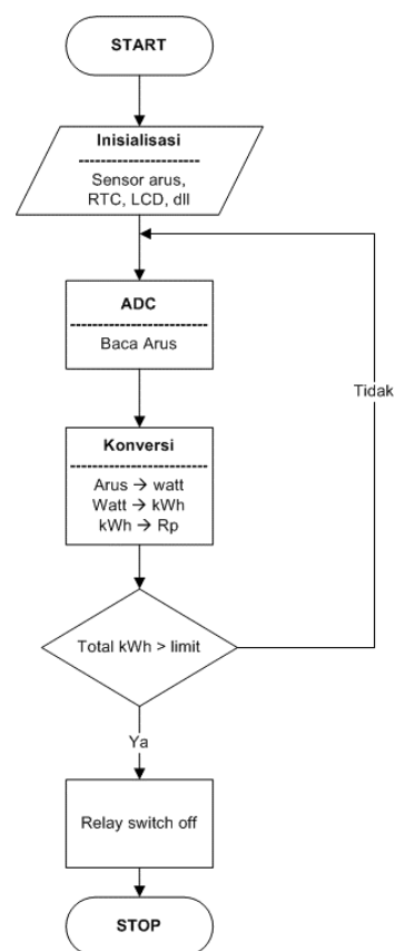
Gambar 6. Flowchart alat ukur konsumsi energi listrik
