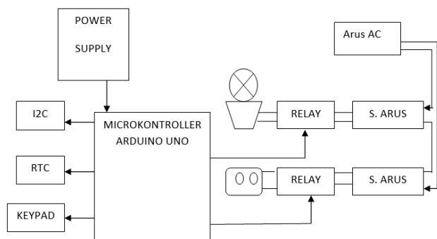
Gambar 5. Diagram blok sistem alat ukur konsumsi listrik
