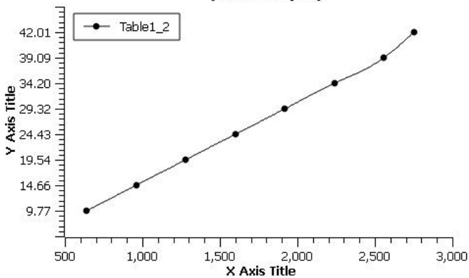
Gambar 8. Grafik daya listrik dihasilkan angin
