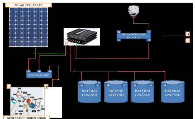
Gambar 6. Rangkaian percobaan
