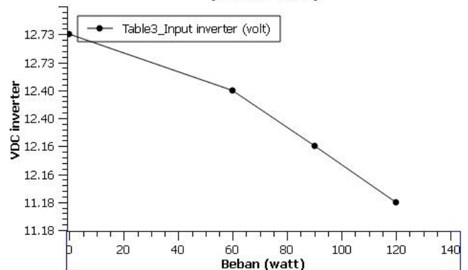
Grafik perubahan Vin inverter terhadap beban (volt vs watt)
