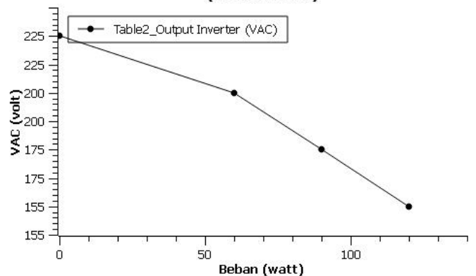
Gambar 10. Grafik perubahan tegangan terhadap beban pada inverter
