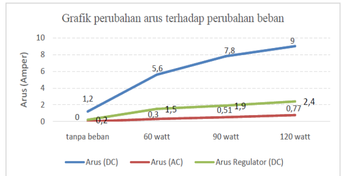
Gambar 9. Grafik perubahan arus terhadap perubahan beban
