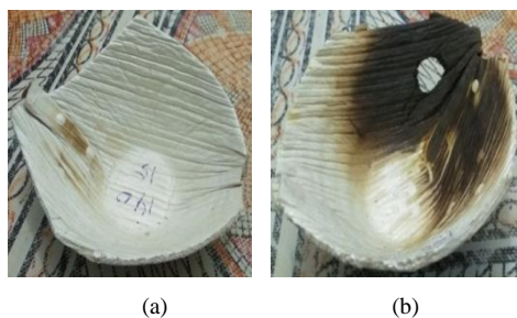
Gambar 2. Karakteristik permukaan atas hasil pengepresan dengan temperatur: (a) 140 °C, dan (b) 150 °C
