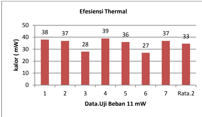
Gambar 6. Efisiensi thermal pada beban 11 MW
