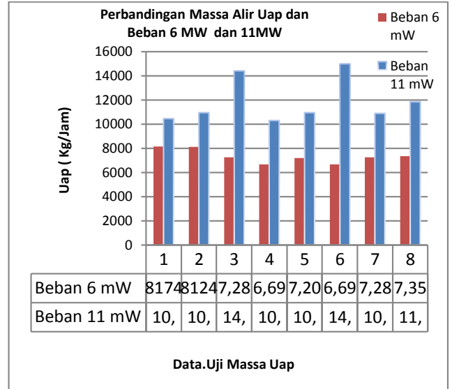
Gambar 7. Perbandingan Massa uapbeban 6 MW dan 11 MW
