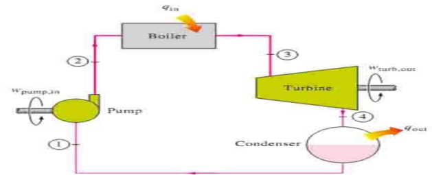
Gambar.2.2 Siklus Rankine
