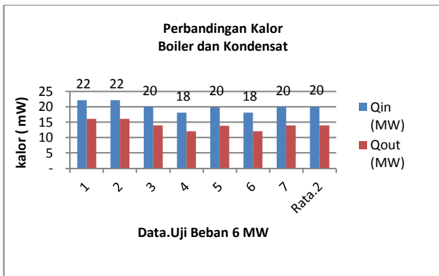
Gambar. Laju heat transfer pada beban 6 MW
