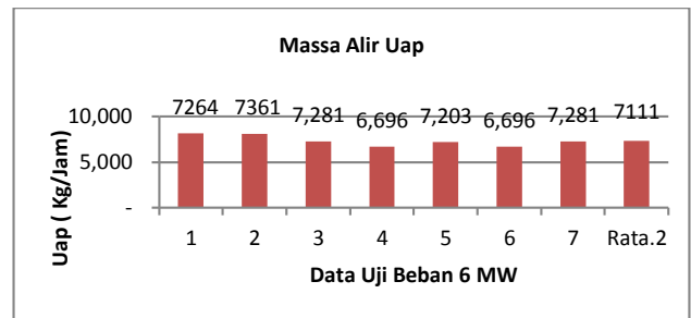
Gambar 4.1. Massa Uap yang mengalir pada beban 6 MW
