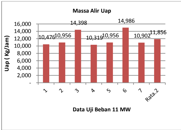
Gambar 4. Massa Uap yang mengalir pada beban 11 MW
