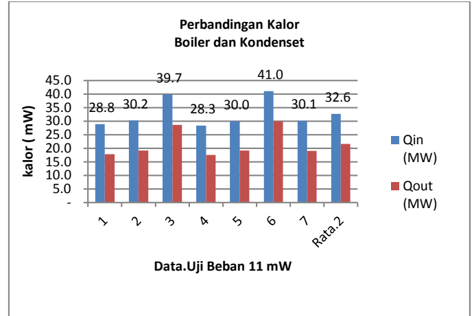
Gambar 5. Laju heat transfer pada beban 11 MW
