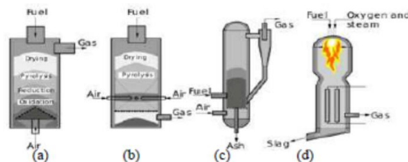
Gambar 1. Tipe Gasifier berdasarkan Arah Aliran, (Hantoko dkk, 2014)
