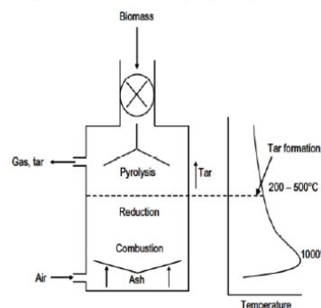
Gambar 4 Zona Reaksi Gasifikasi
