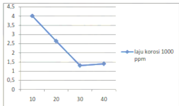
Gambar 4. Grafik Laju Korosi Pada Konsentrasi 1000ppm
