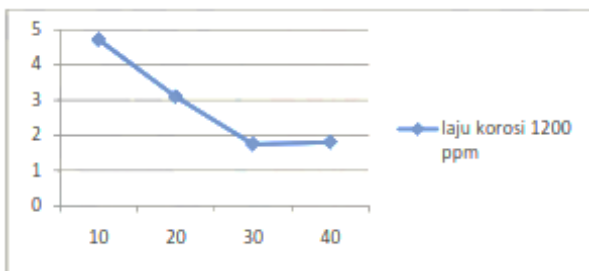
Gambar 5. Grafik Laju Korosi Pada Konsentrasi 1200ppm
