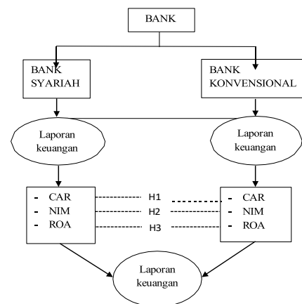
Gambar 1. Kerangka Konseptual
