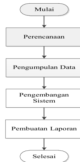
Gambar 2. Kerangka Kerja
